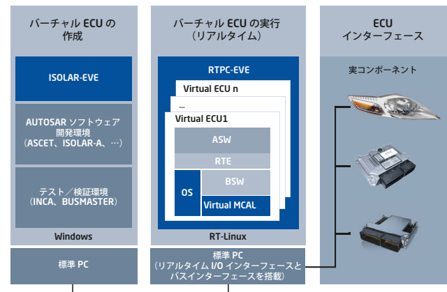
図 1：ISOLAR-EVE を使用したバーチャル ECU
