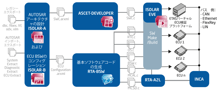
図 2：ETAS の AUTOSAR ソリューション
