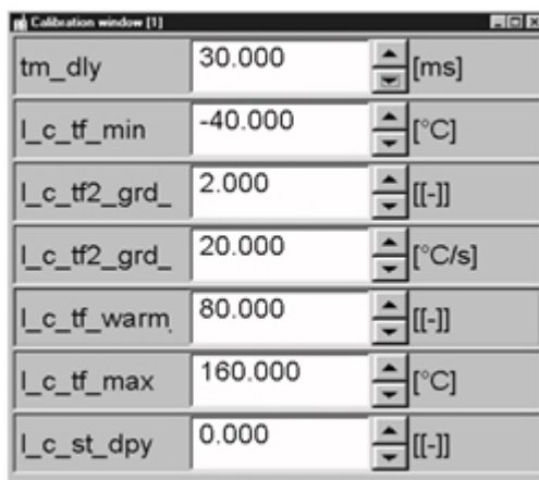
Fig. 2-6: Editeurs de paramètres à l'état hors ligne
