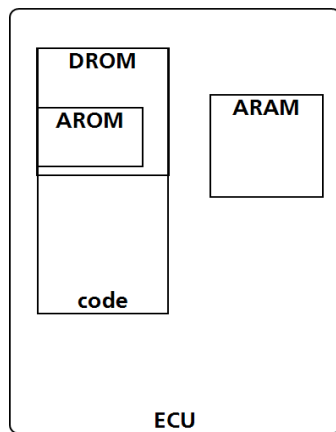
Fig. 1-1: Segmentation mémoire dans le cas de la procédure de calibration InCircuit2
