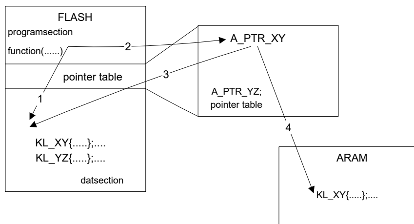
Fig. 1-2: Processus InCircuit2 dans l'ECU
