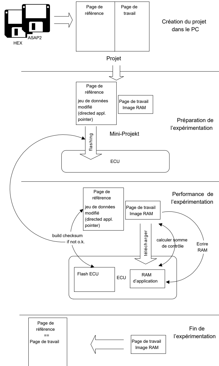
Fig. 1-3: Déroulement schématique de la procédure InCircuit2 dans INCA
