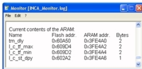
Fig. 2-2: Paramètres actuellement sélectionnés avec adresses mémoire
